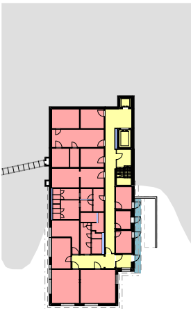
2. Untergeschoss
