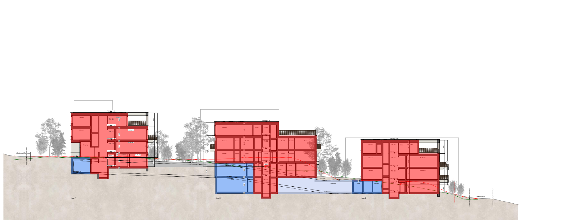
Längsschnitt 3-3
