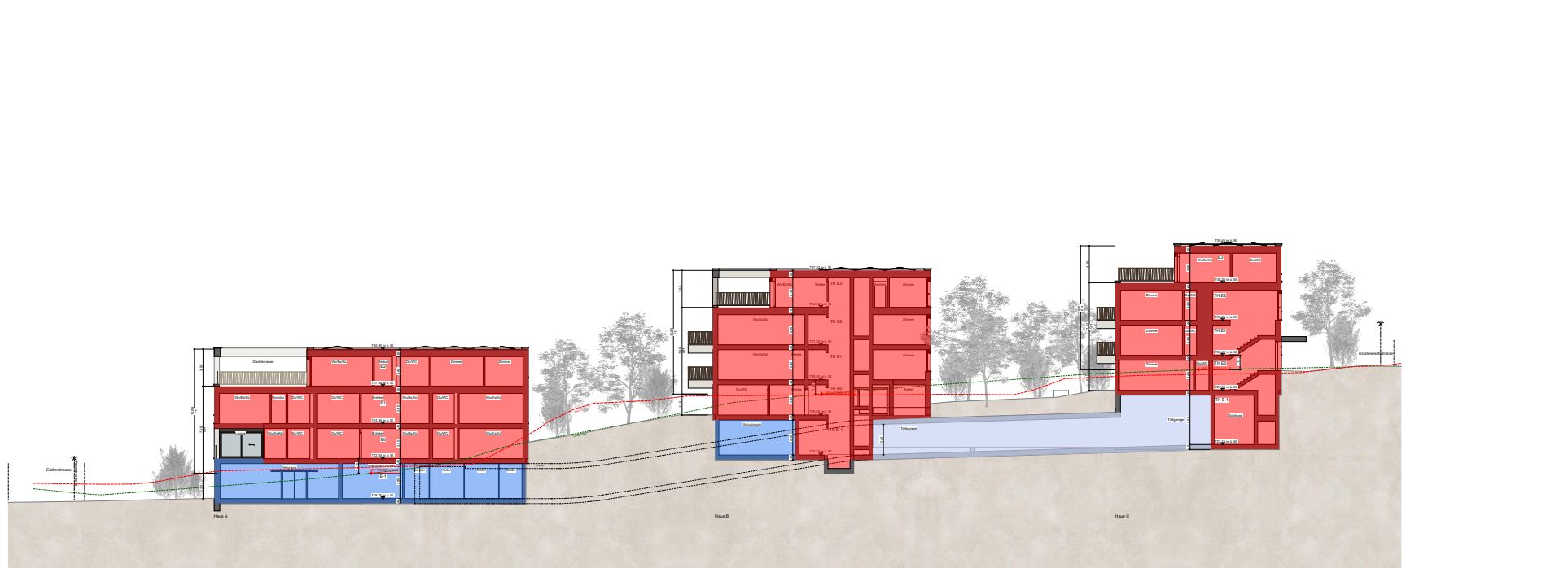
Längsschnitt 1-1
