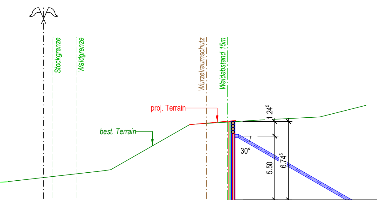
Profil 6-6, 1:200
