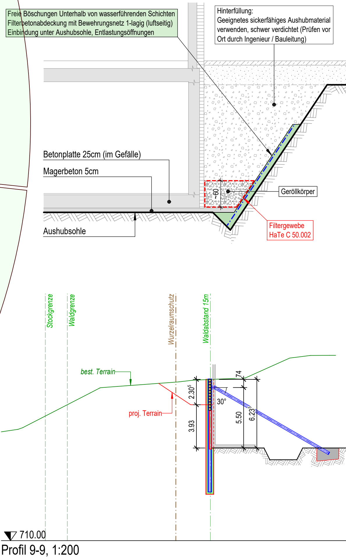
Schemaschnitt 1:50 Sohle, Böschungssicherung, Hinterfüllung
