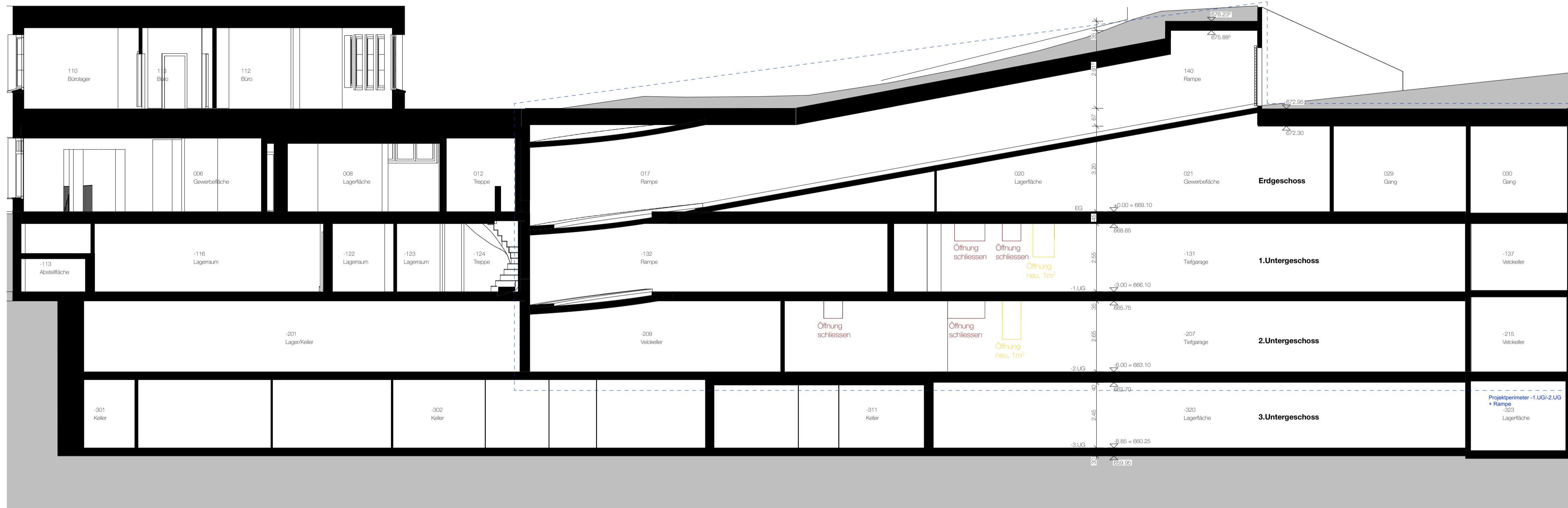
Schnitt 01
