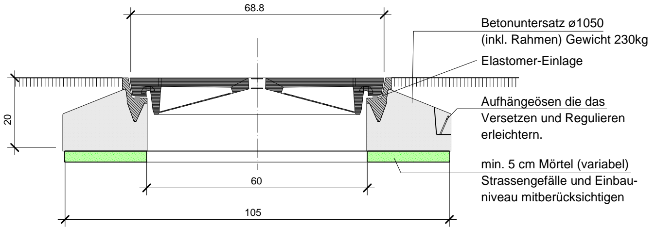
Schachtabdeckung von Roll Fig.2633.010.10 (D400)K
