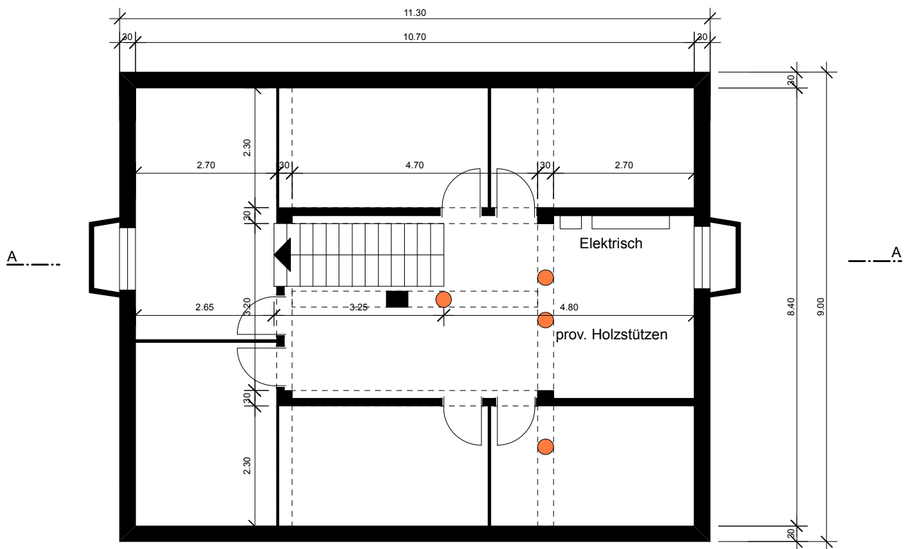
Grundriss
